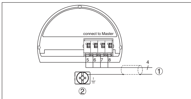
Fig. 26: Wiring plan CPT-2x Slave sensor
